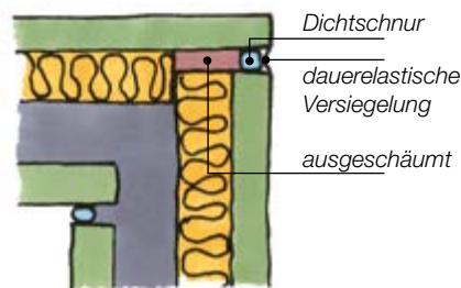
Draufsicht Wanddeckausbildung
