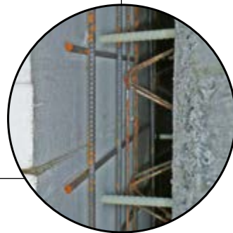
Schöck Thermoanker
